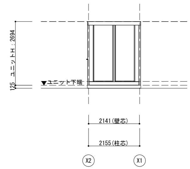
Y2通り立面図
