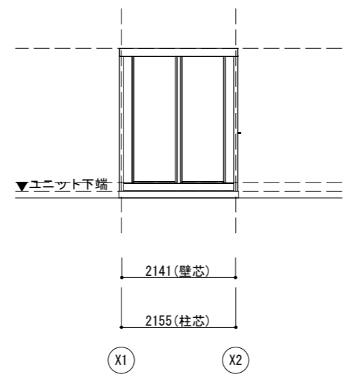
Y1通り立面図
