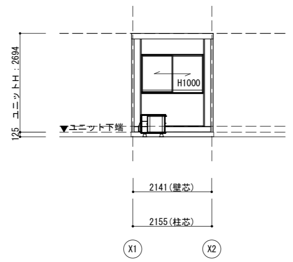
Y1通り立面図
