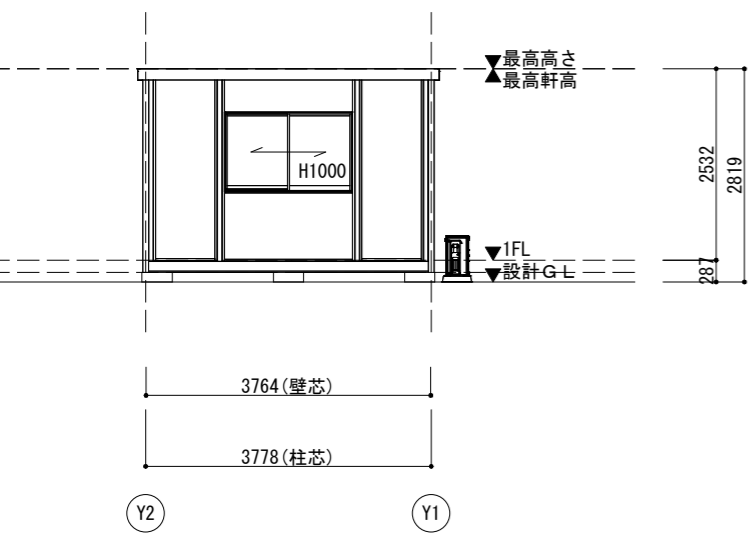
X1通り立面図
