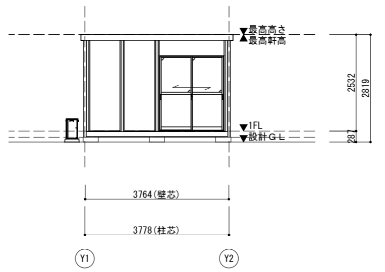
X2通り立面図
