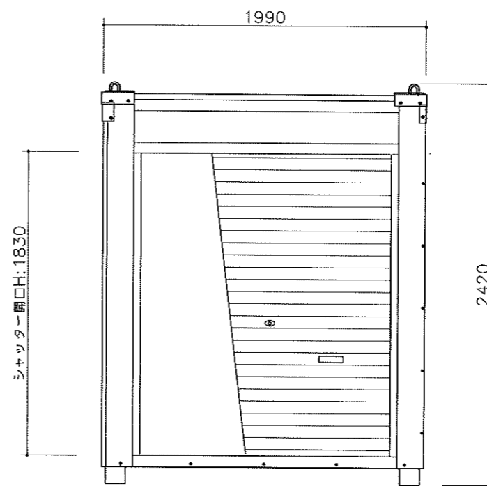
X1通り立面図
