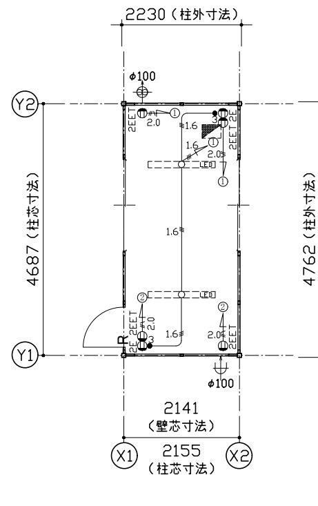
電気配線図
