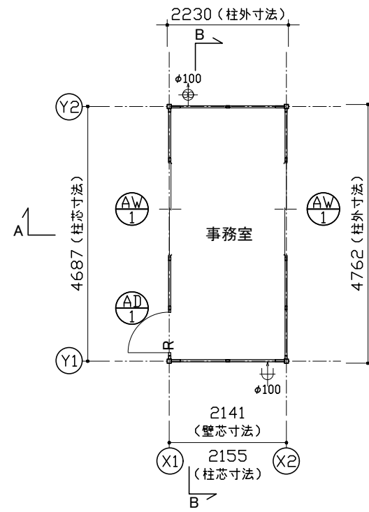
平面図
